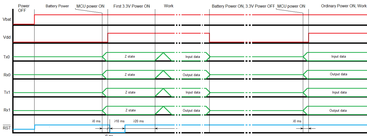
Рис. 5. Временная диаграмма состояний и уровней сигналов на выводах модуля при применении Vbat.
