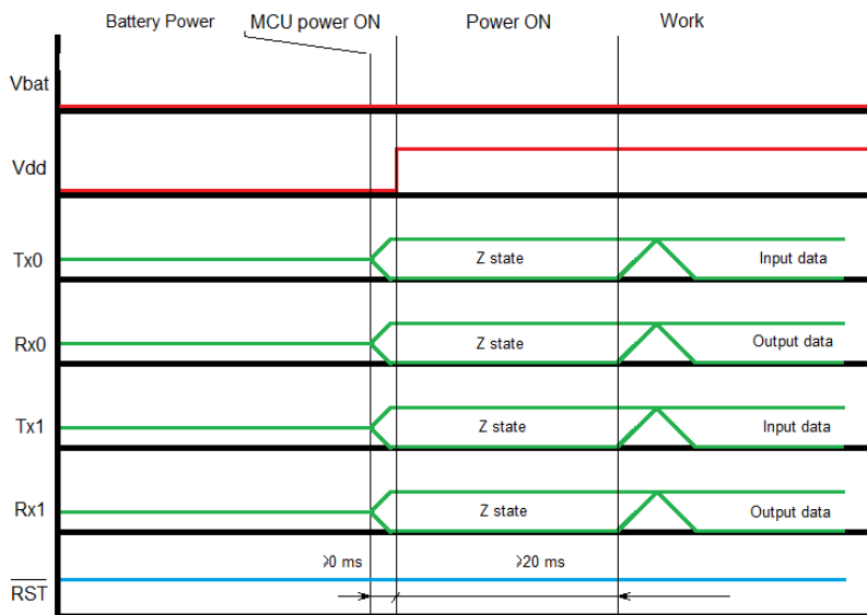
Рис. 6. Временная диаграмма состояний и уровней сигналов на выводах модуля при применении модуля без Vbat.
