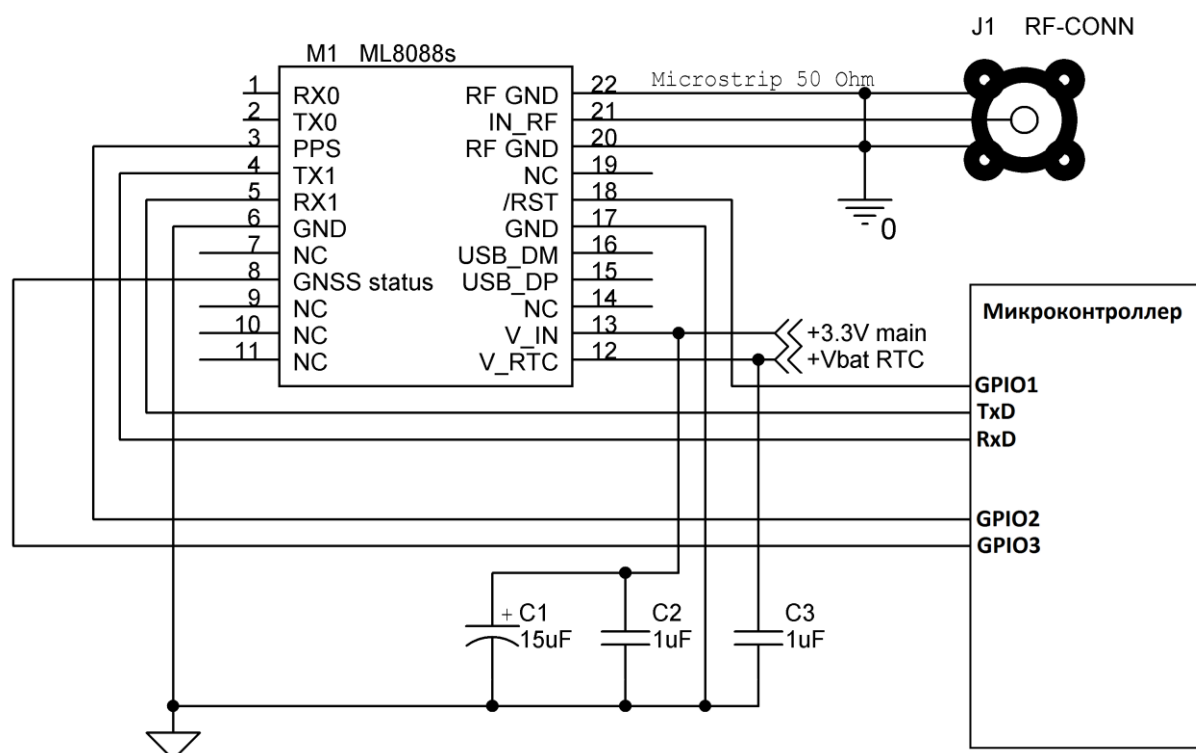
Рис.4. Типовая схема включения приемника ML8088s с передачей данных NMEA по UART1.
