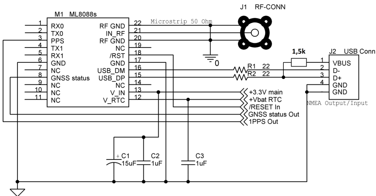
Рис.7. Типовая схема включения приемника ML8088s с передачей данных NMEA по USB.
