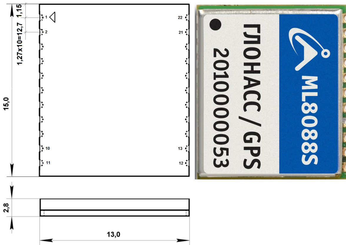
Рис.2. Габаритно-присоединительные размеры приемника ML8088s. Контактные площадки показаны пунктирной линией. Номера контактов и метка первого вывода показаны условно.
