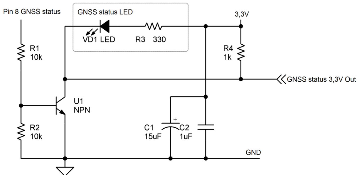
Рис.8. Типовая схема преобразования выходного уровня сигнала GNSS status приемника ML8088s и подключения индикаторного светодиода.
