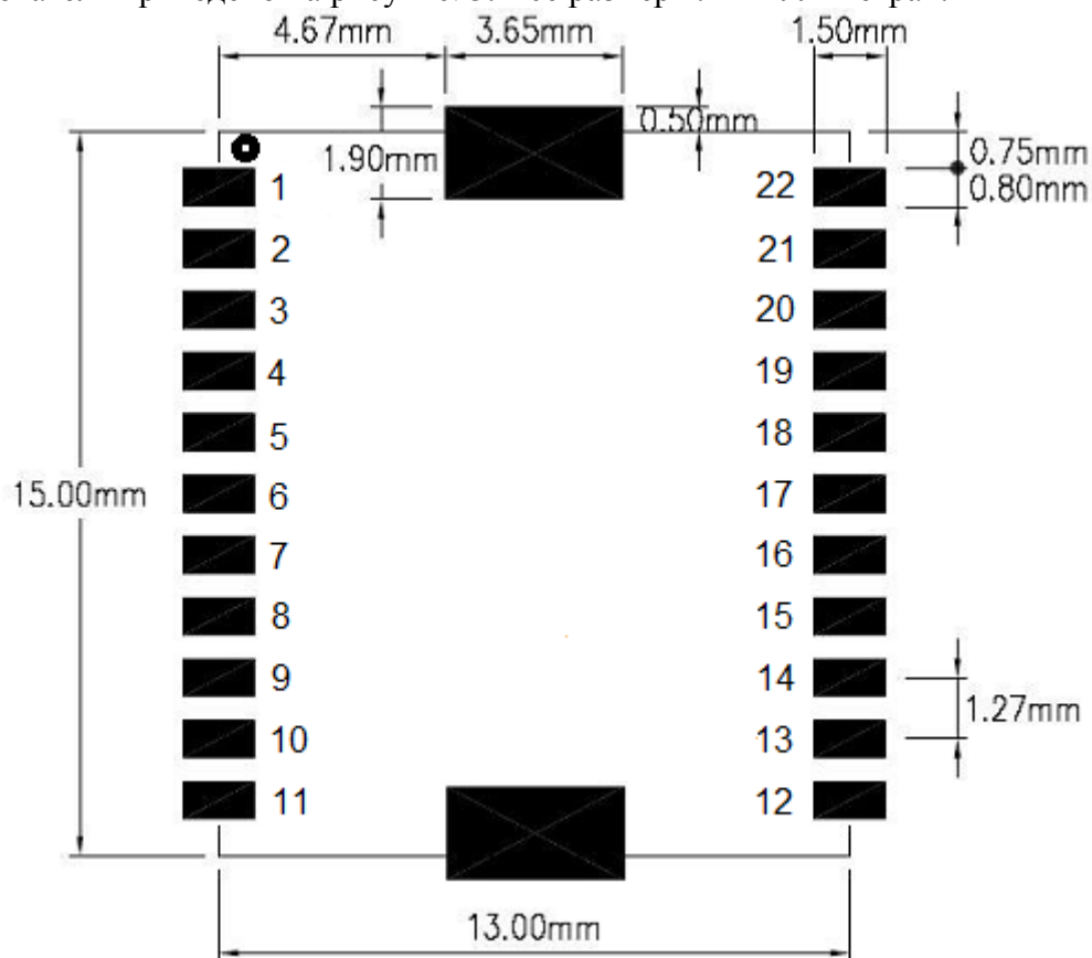
Рис.3. Рекомендуемое посадочное место для установки приемника ML8088s. Номера выводов и метка первого вывода показаны условно.
